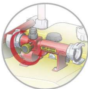
Livré avec proportionneur "MIXY EDUCTOR" 200 ou 400 L/min, avec soupape de régulation et robinet doseur
